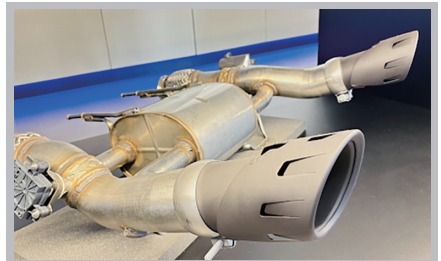
⑥ マフラー ・ASSY MUFFLER AND TAILPIPE-SPT 限定1セット / ¥ 950,000 約 9 万円お得
